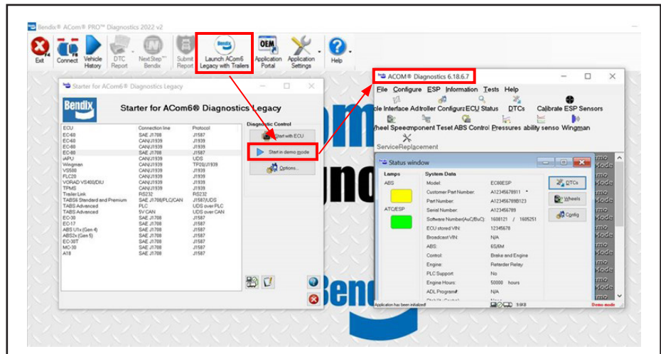
Figura 2 - Identificación de la versión del software ACom 6 Legacy
