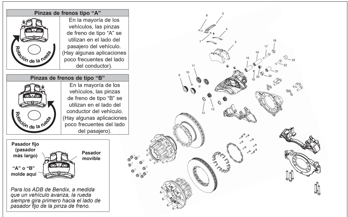
Figura 1 - Frenos de disco neumático (ADB) Bendix® SB-7™ y Bendix® SN-7™
