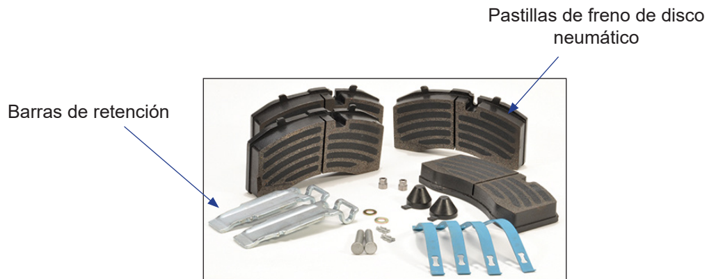
Contenido del juego de pastillas ADB22X® de Bendix® n.º de pieza K182236
