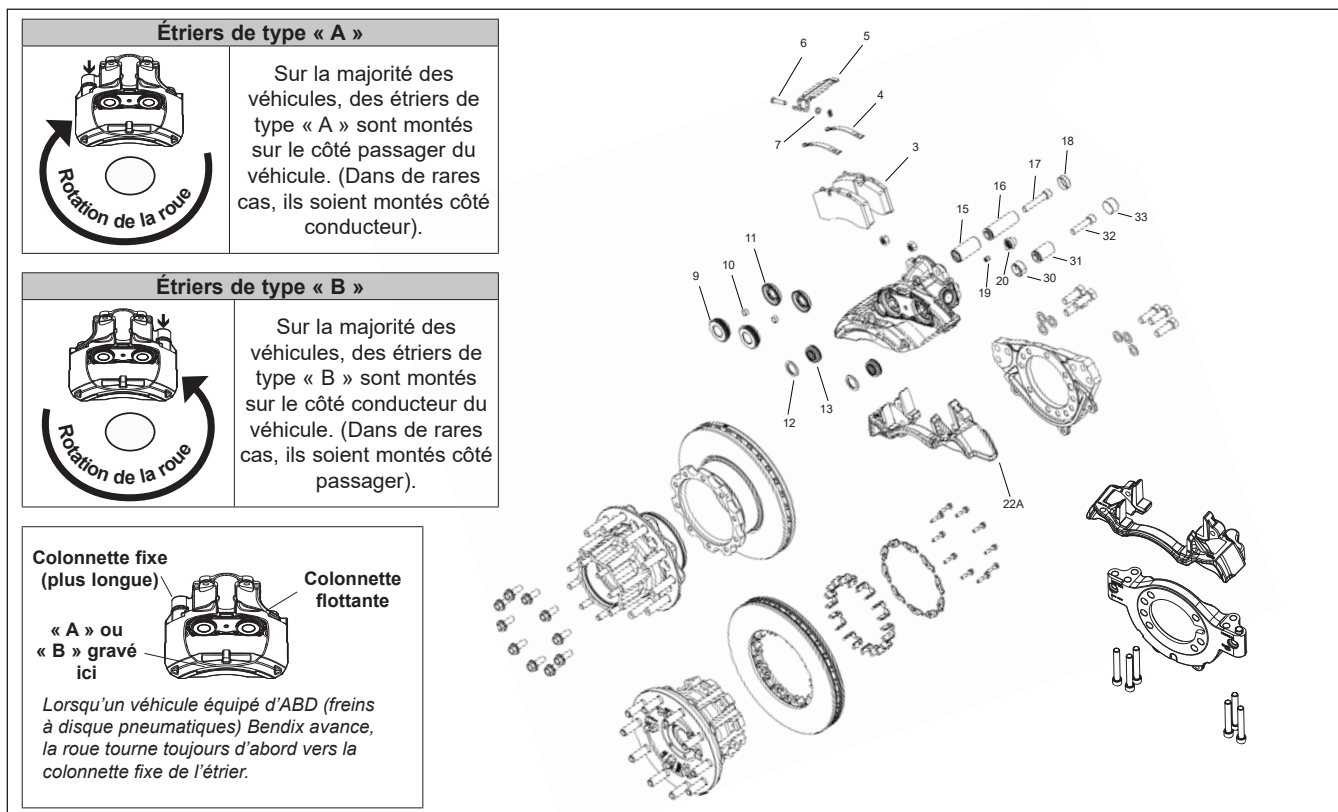
Figure 1 - Freins à disque pneumatiques (ADB) Bendix® SN-6™ et SN-7™
