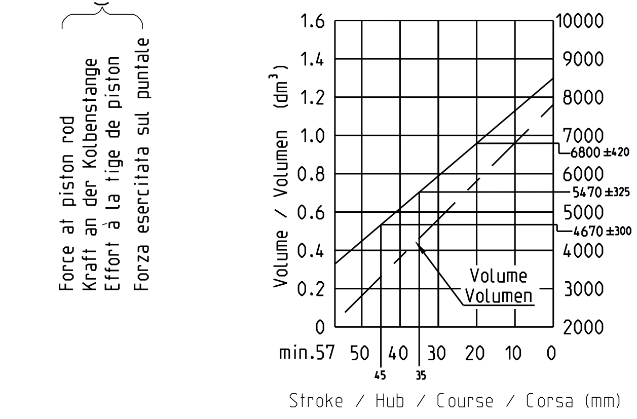
Force at piston rod Kraft an der Kolbenstange Effort à la tige de piston Forza esercitata sul puntale
