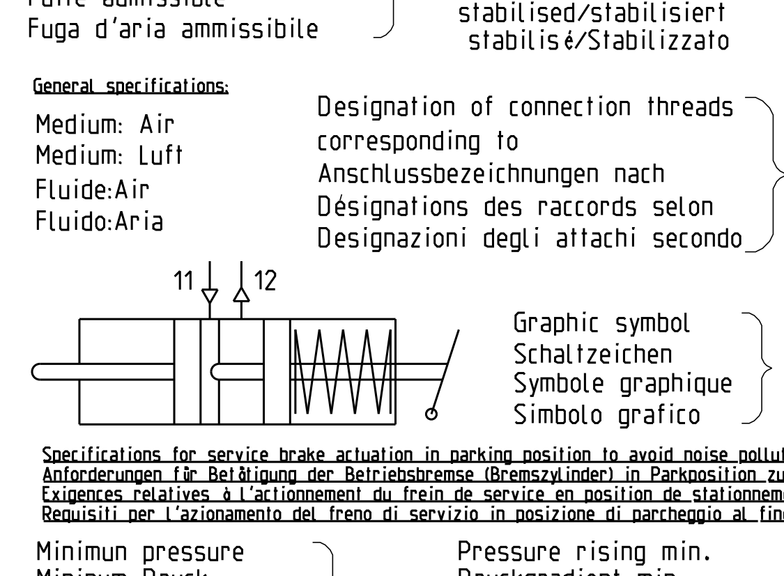
Breather hole opened Atmungsböhrung geöffnet Trou de respiration ouvert Foro di respirazione aperto
