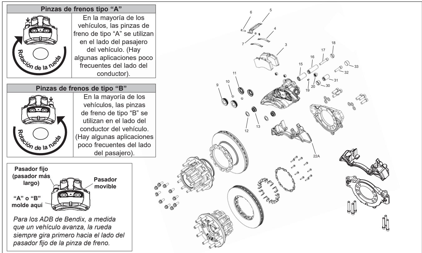
Figura 1: freno de disco neumático (ADB) Bendix® SN-6™
