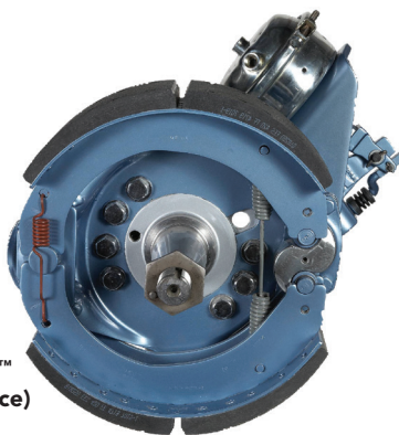
Bendix® Versajust® Automatic Slack Adjuster
